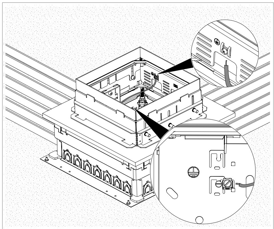
Fig. 10: Creating the equipotential bonding
